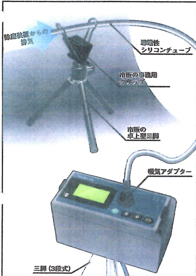
■設置例1 アルミダクト内に粉じん計への空気取り込み配管を入れる
