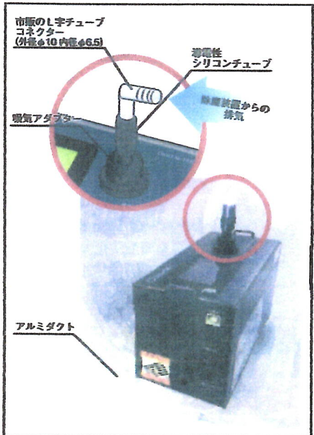
■設置例2 アルミダクトの中に粉じん計を設置
